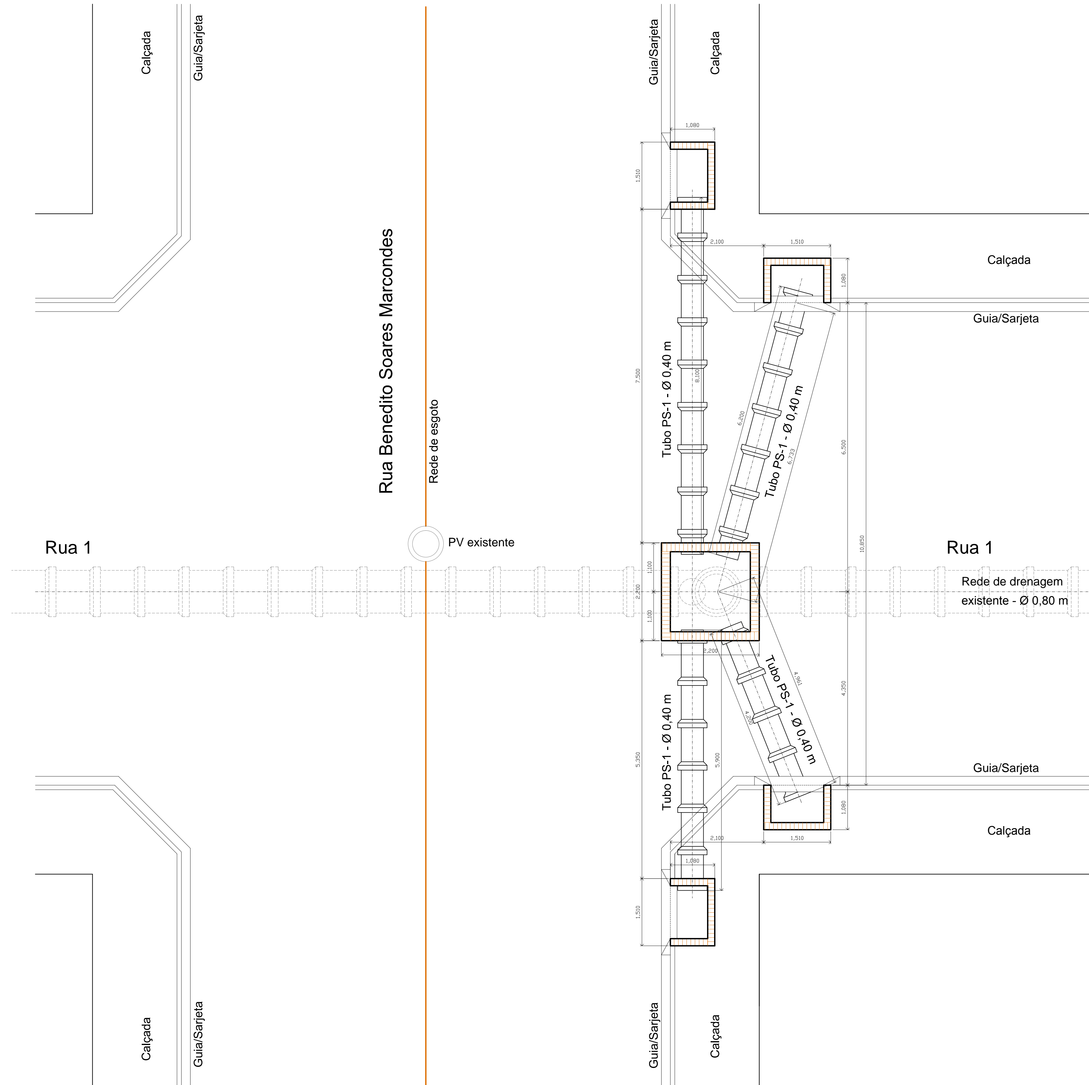
PLANTA BAIXA - POÇO DE VISITA E BOCA DE LOBO 1 : 50
