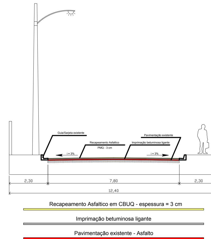
Perfil Transversal da Rua Ver. Lázaro Gazeta
