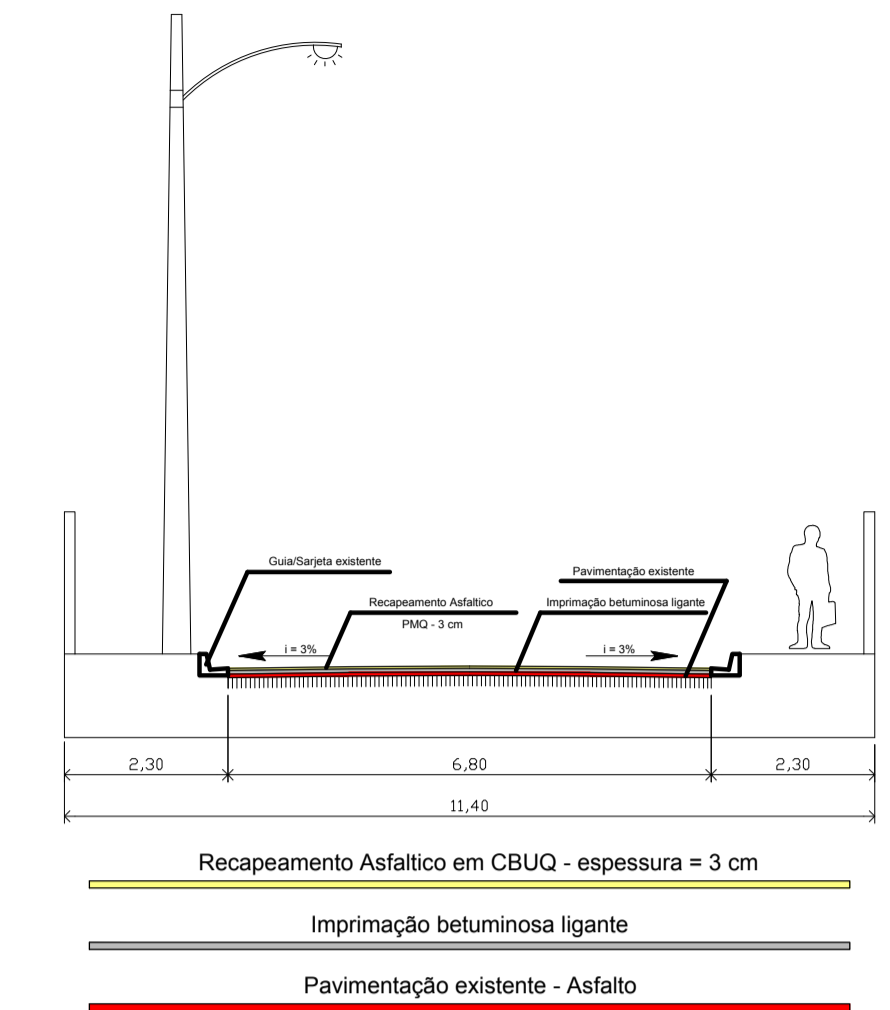
Perfil Transversal da Rua Francisco Mattos
