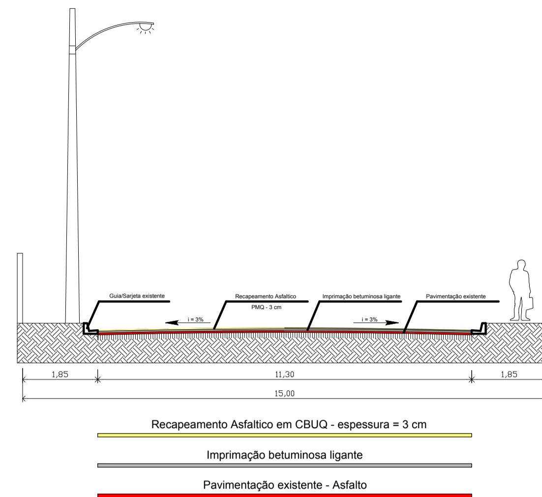
Perfil Transversal da Rua Paulo de Azevedo
