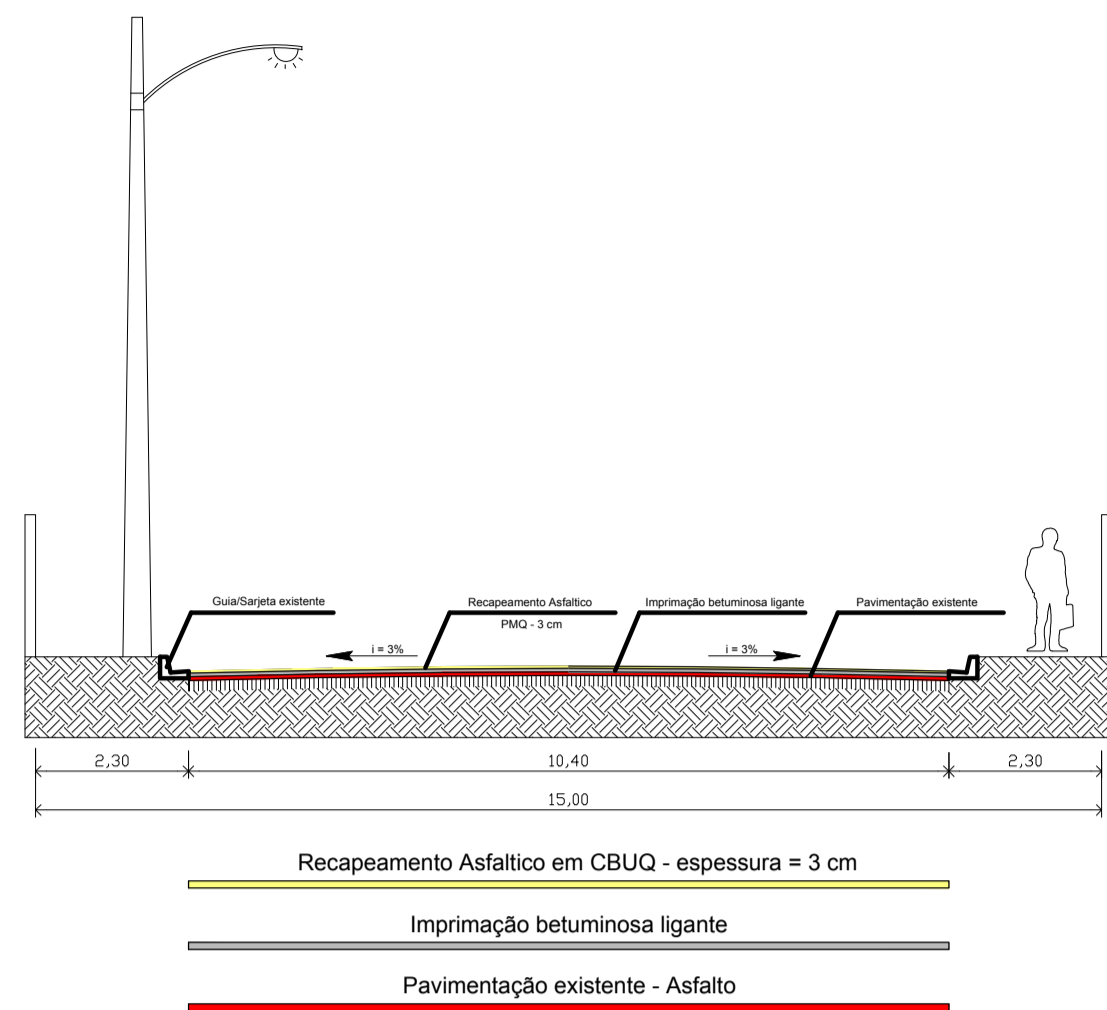
Perfil Transversal das Ruas Benedito S. Marcondes, Correia de Menezes, José Maria Mathias, Brasília e Curitiba
