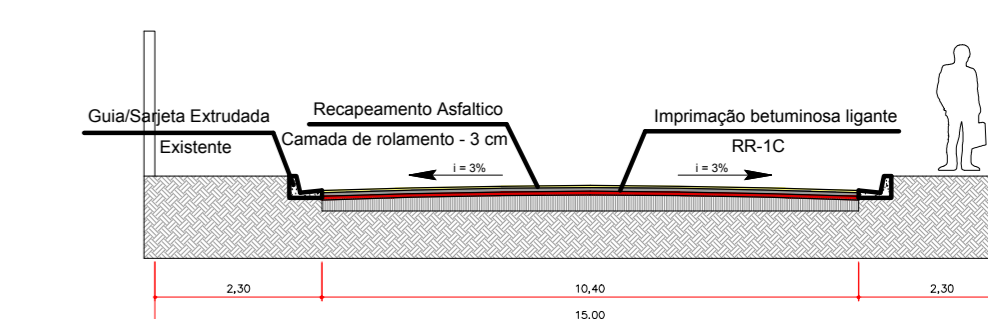
Recapeamento asfáltico - e = 3 cm Imprimação betuminosa ligante - RR-1C Pavimentação existente - Asfalto Perfil - Recapeamento Asfáltico Benedito S. Marcondes e Correia de Menezes
