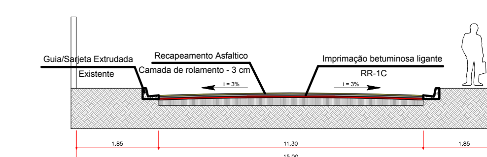
Recapeamento asfáltico - e = 3 cm Imprimação betuminosa ligante - RR-1C Pavimentação existente - Asfalto Perfil - Recapeamento Asfáltico - Rua Paulo de Azevedo
